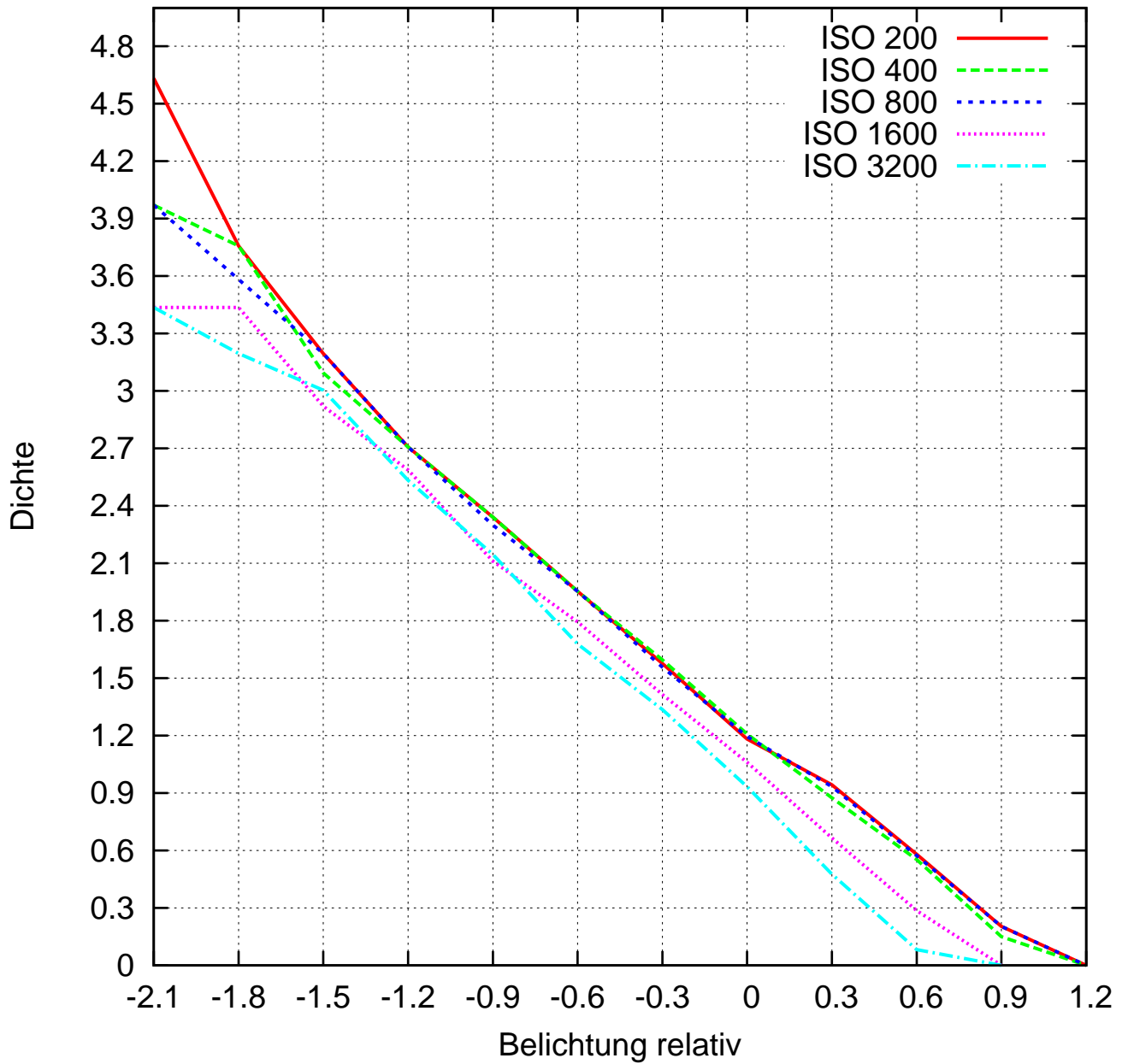
Belichtungskurven Nikon D 300
